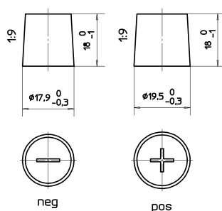
Anschlusspole 1
